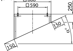
Наклонный крышный цоколь
