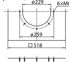
Присоединительный фланец
