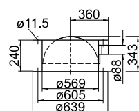
ZLK 21-0560 Моторизированный запорный клапан
