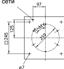
Подключение DV 30-25 к сети
