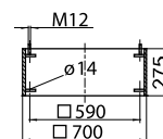
Прокладка
