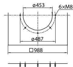
Фланец присоединения
