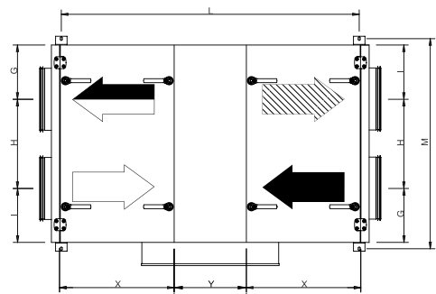
Правостороннее исполнение
