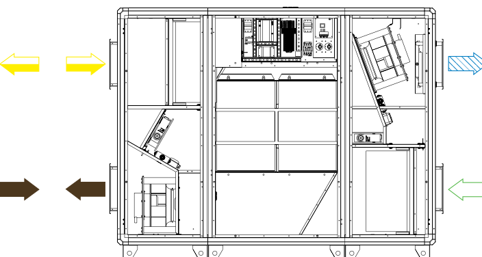
Правосторонний агрегат
