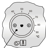
Отверстие контрольной кнопки STB
